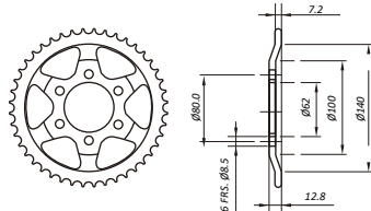
YA07.5_428 XT225 SEROW 1KH
